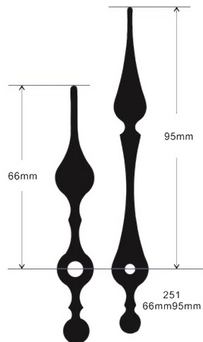
尺寸从中心量起(如图所示)
